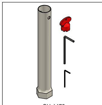
SH-1478 Kit de Llaves de Mantenimiento Maintenance Keys Kit
