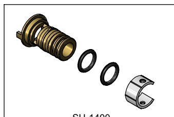
SH-1400 Inserto con O'ring Insert with O'ring
