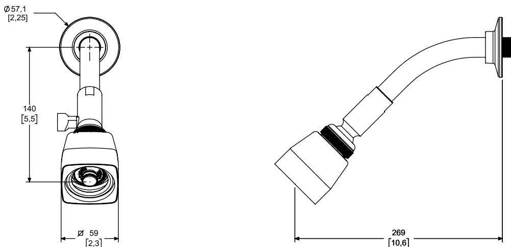
Medidas Referenciales / Estimated Dimensions, Acot. mm [pulg.] / Dim. mm [inch.]
