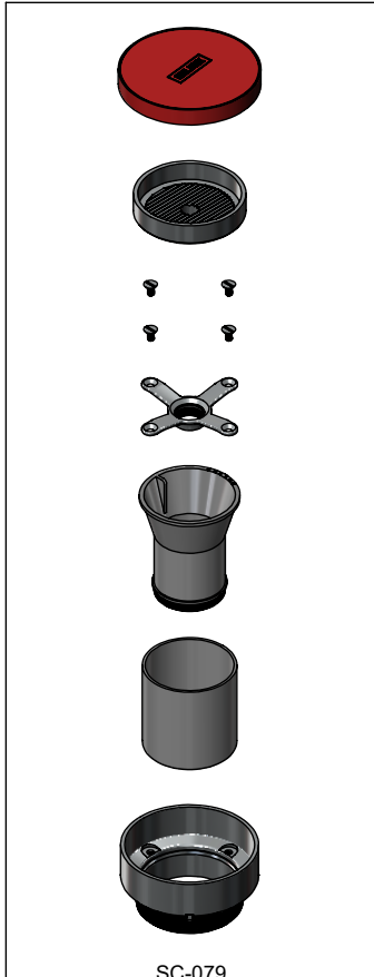
Sub ensamble Contra con Porta Inserto Floor Drain Strainer Kit
