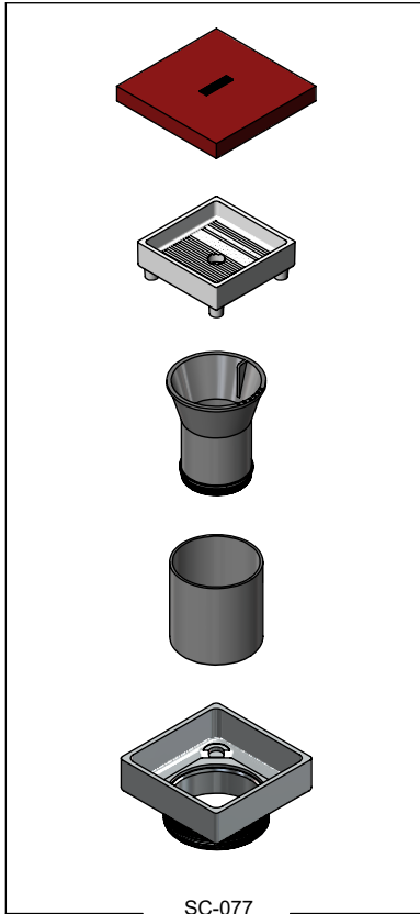
Sub ensamble Contra con Porta Inserto Floor Drain Strainer Kit
