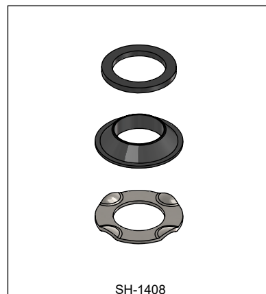
SH-1408 Kit Empaques de Sujeción para Monomando Valve Mounting Kit
