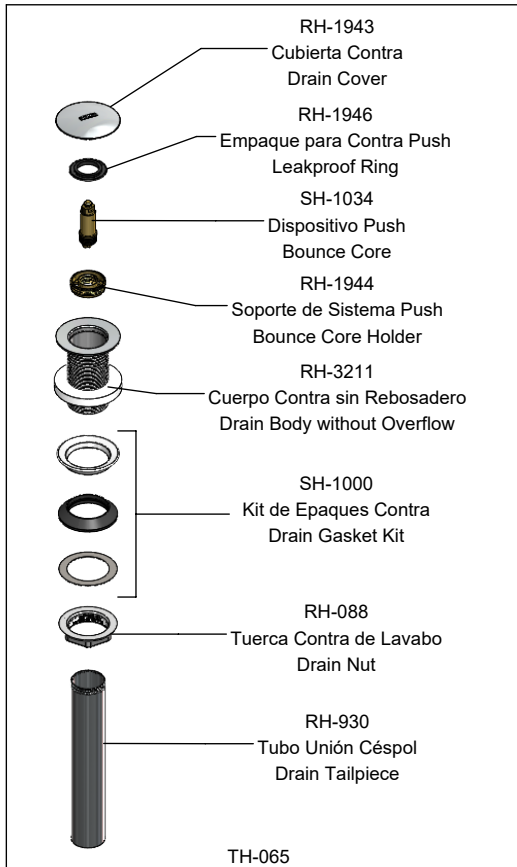
Contra de Push para Lavabo sin Rebosadero Lavatory Push Drain without Overflow
