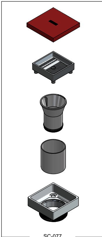
Sub ensamble Contra con Porta Inserto Floor Drain Strainer Kit
