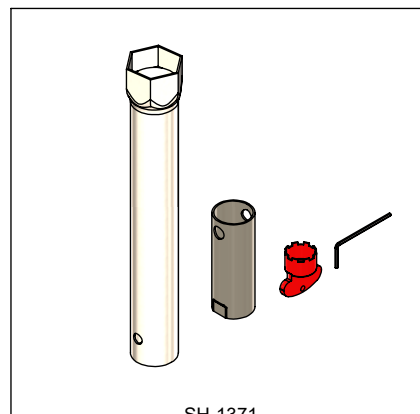
SH-1371 Kit de Llaves de Mantenimiento Maintenance Kit
