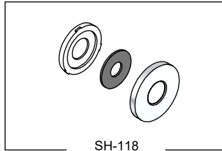
SH-118 Chapetón Armado Assembly Escutcheon
