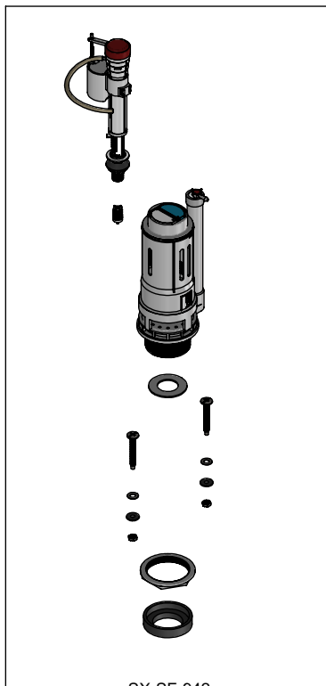
SX-SF-942 Kit Válvula de Admisión y Válvula de Descarga de 3" Fill Valve and 3" Flush Valve Kit
