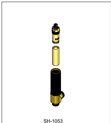
SH-1053 Cuerpo Lateral Izquierdo Armado Valve Left Body
