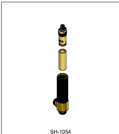
SH-1054 Cuerpo Lateral Derecho Armado Valve Right Body
