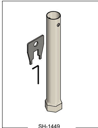
Kit de Mantenimiento Maintenance Kit
