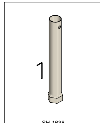
SH-1638 Kit de Llaves de Mantenimiento Maintenance Wrench Kit
