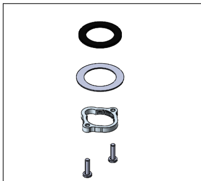
SB-1387 Kit de Sujeción Mounting Kit
