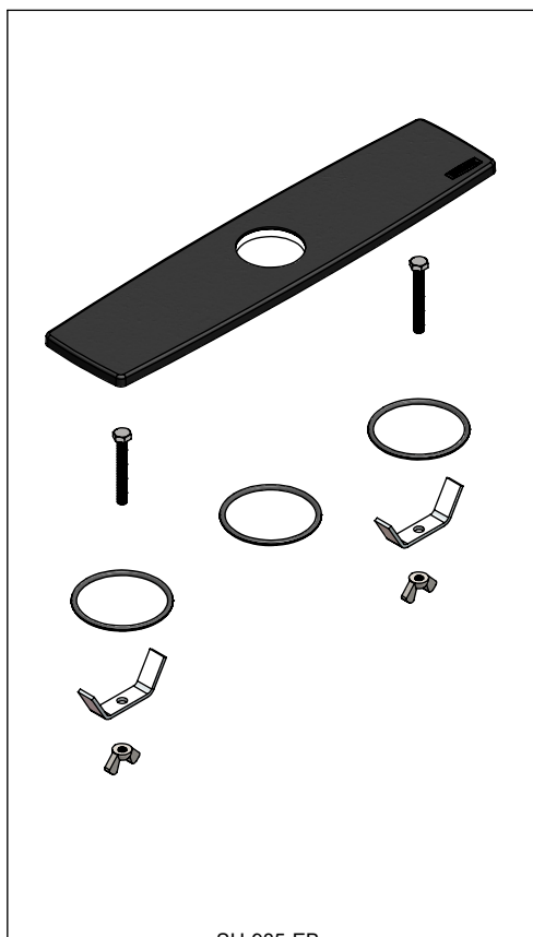
SH-985-EB Chapetón Cubre Taladros Hole Cover Escutcheon
