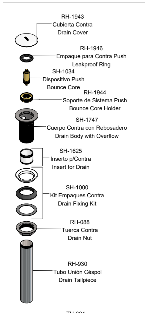
Contra de Push para Lavabo sin Rebosadero Push Drain Lavatory without Overflow
