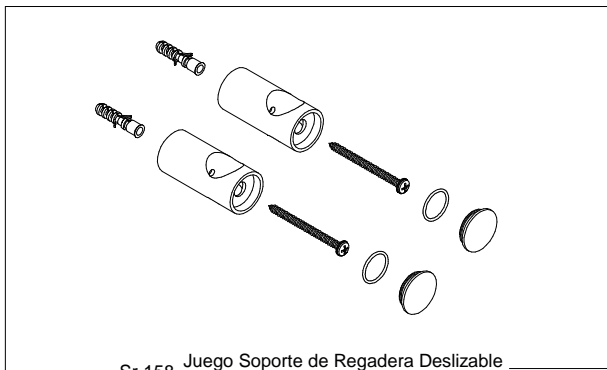
Sr-158 Juego Soporte de Regadera Deslizable Sliding Shower Game Support
