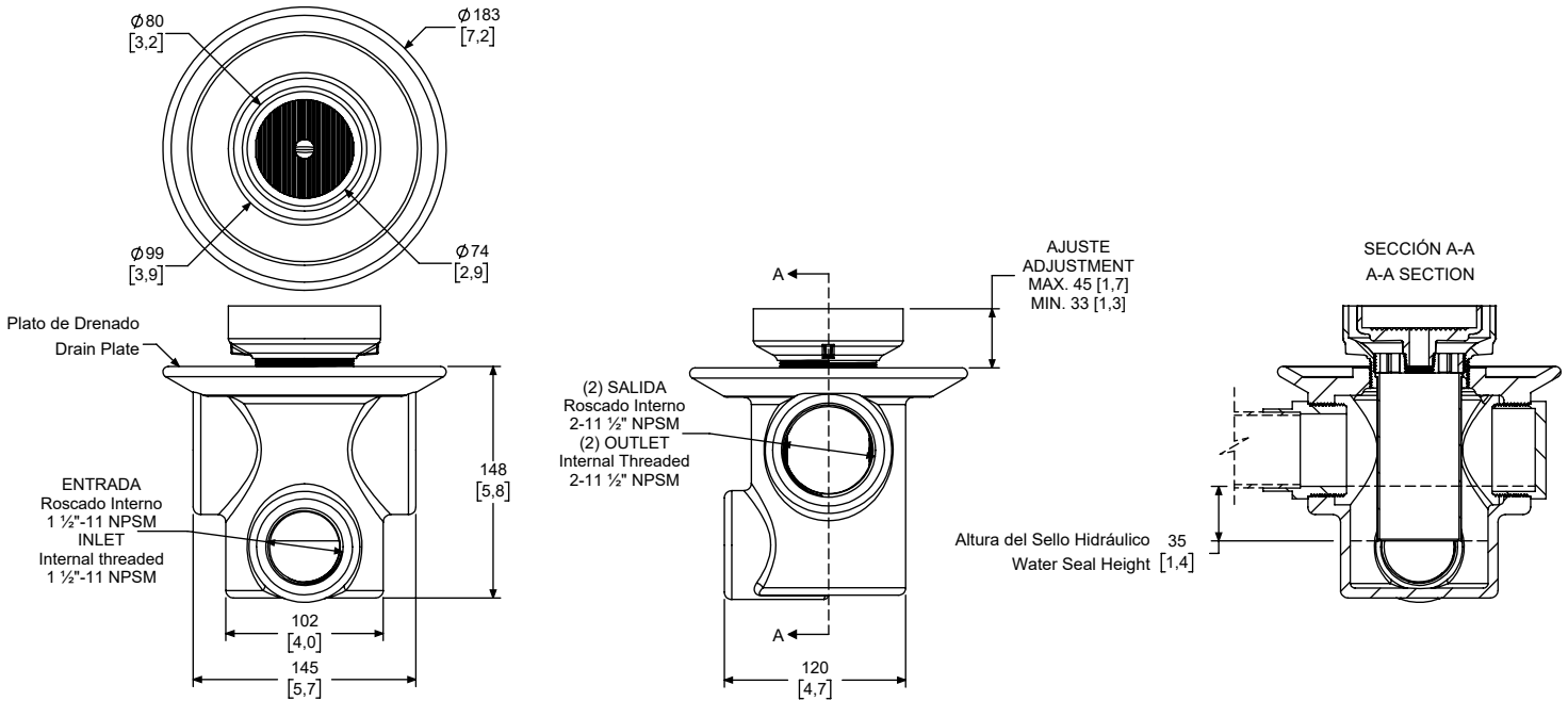
Medidas Referenciales / Estimated Dimensions, Acot. mm [pulg.] / Dim. mm [inch.]
