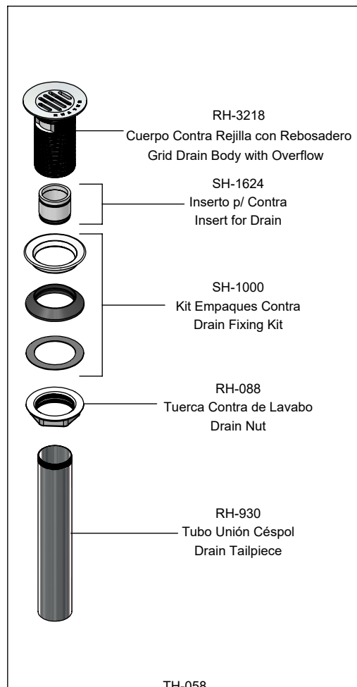
TH-058 Contra con Rejilla para Lavabo con Rebosadero Lavatory Sink Grid Drain with Overflow
