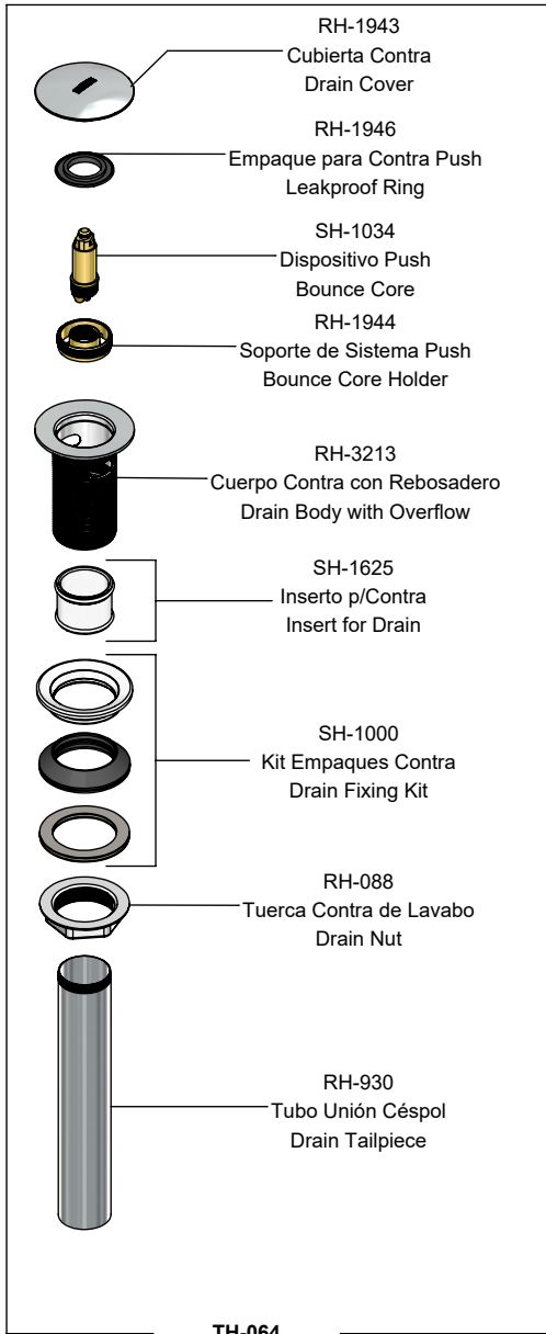
TH-064 Contra de Push para Lavabo sin Rebosadero Push Drain Lavatory without Overflow
