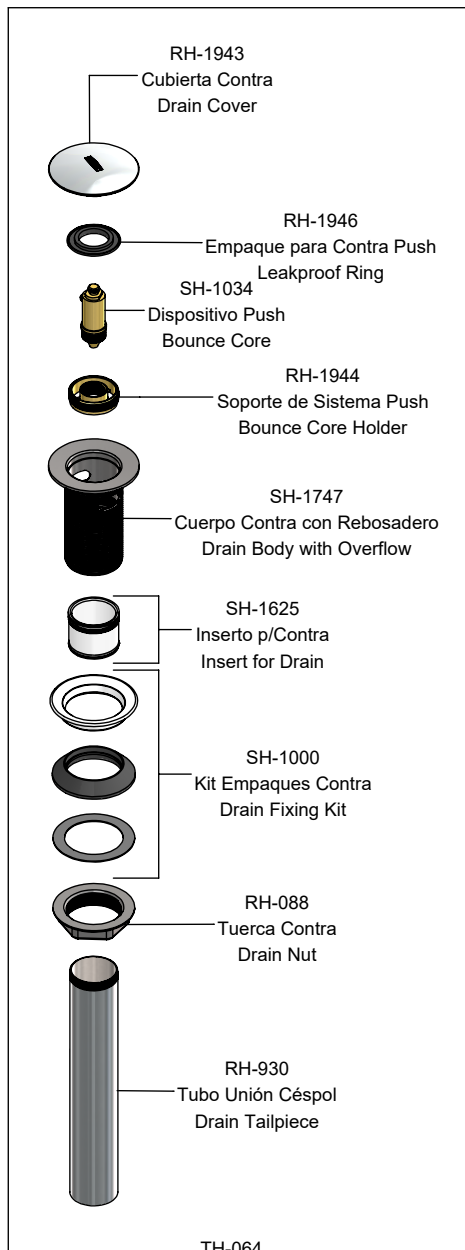
TH-064 Contra de Push para Lavabo sin Rebosadero Push Drain Lavatory without Overflow
