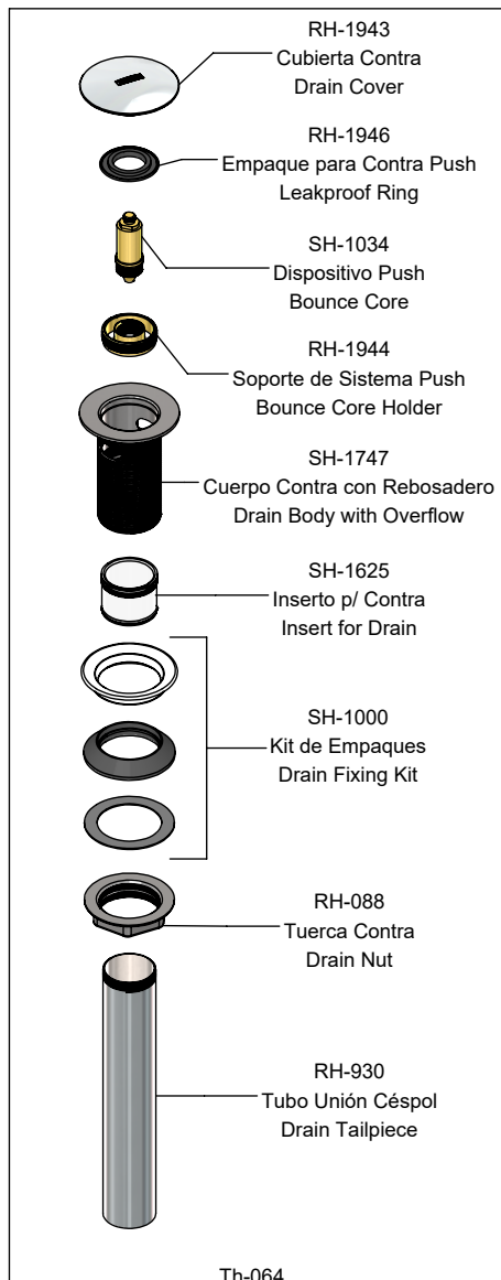
Th-064 Contra de Push para Lavabo sin Rebosadero Push Drain Lavatory without Overflow
