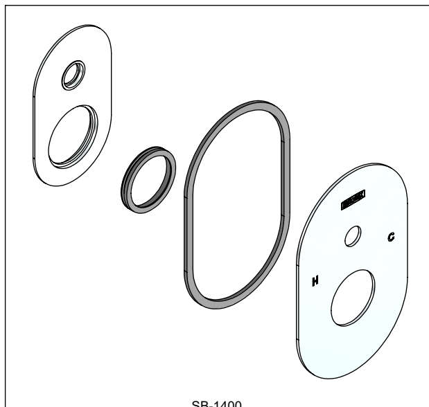
SB-1400 Kit Chapetón Escutcheon Kit
