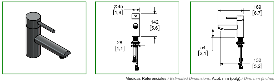
Medidas Referenciales / Estimated Dimensions. Acot. mm (pulg.) / Dim. mm (inches).
