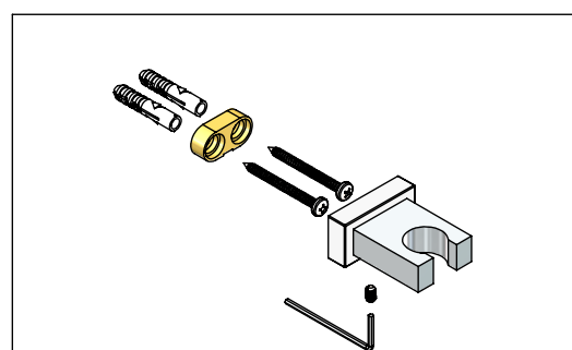
Soporte para Regadera Holder for Shower
