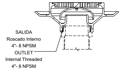
SECCIÓN A-A A-A SECTION
