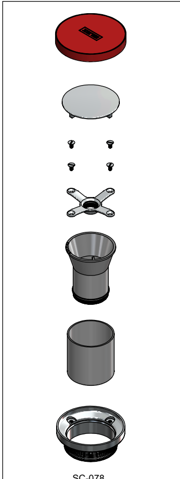
Sub ensamble Contra con Cúpula Floor Drain Strainer Kit
