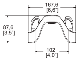
Dimensiones: vista frontal
