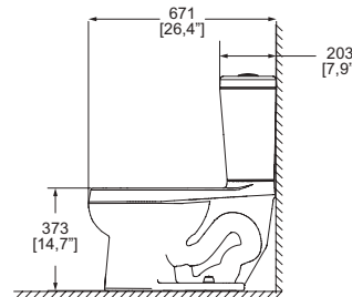
Dimensiones: vista lateral
