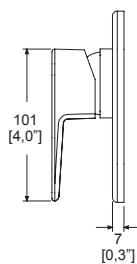
Dimensiones: vista lateral
