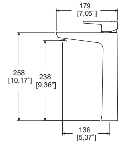
Dimensiones: vista lateral
