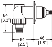
Dimensiones: vista lateral
